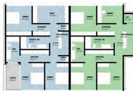
Grundriss Obergeschoss
