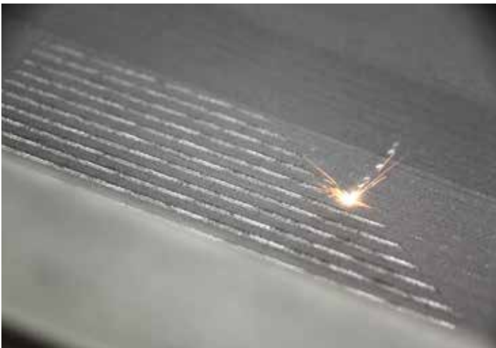
Der Laser der 3Dmetalprinting Maschine baut schichtweise Metall zu komplexen Konstruktionen auf.
